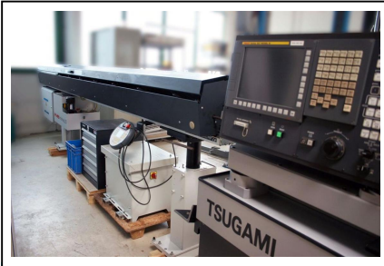
Langdrehautomat
