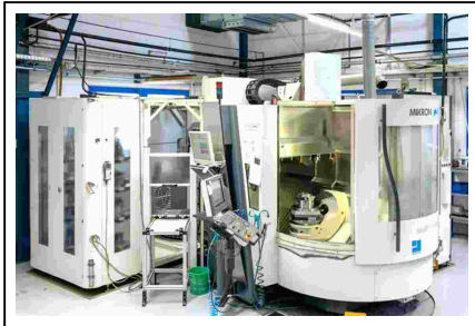
Bearbeitungszentrum - Universal MIKRON HSM 600 U ProdMod Nr. 1032-03888 Baujahr 2005 x-Weg 800 mm y-Weg 600 mm z-Weg 500 mm
