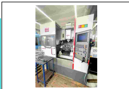
Bearbeitungszentrum - Universal QUASER UX 300/15C Nr. 1032-03866 Baujahr 2011 x-Weg 410 mm y-Weg 610 mm z-Weg 500 mm
