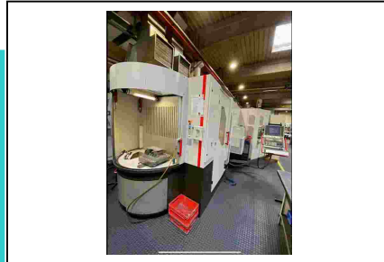
Bearbeitungszentrum - Universal HERMLE C 30 UP Nr. 1032-03877 Baujahr 2010 x-Weg 650 mm y-Weg 600 mm z-Weg 500 mm
